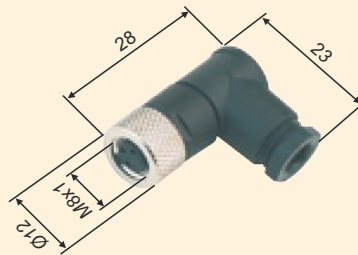
CCP8-3FA-G
