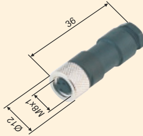
CCP8-3FS-G
